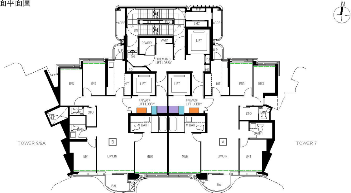
Tower 8 9/F Floor Plan 第8座 9樓樓面平面圖
