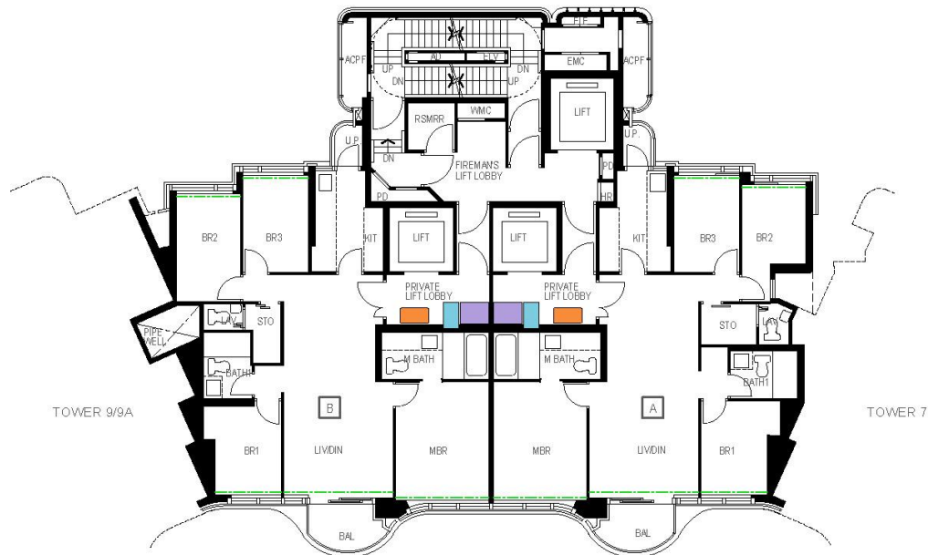
Tower 8 10/F-12/F,15/F-23/F & 25/F-26/F Floor Plan 第8座 10樓至12樓、15樓至23樓及 25樓至26樓 樓面平面圖
