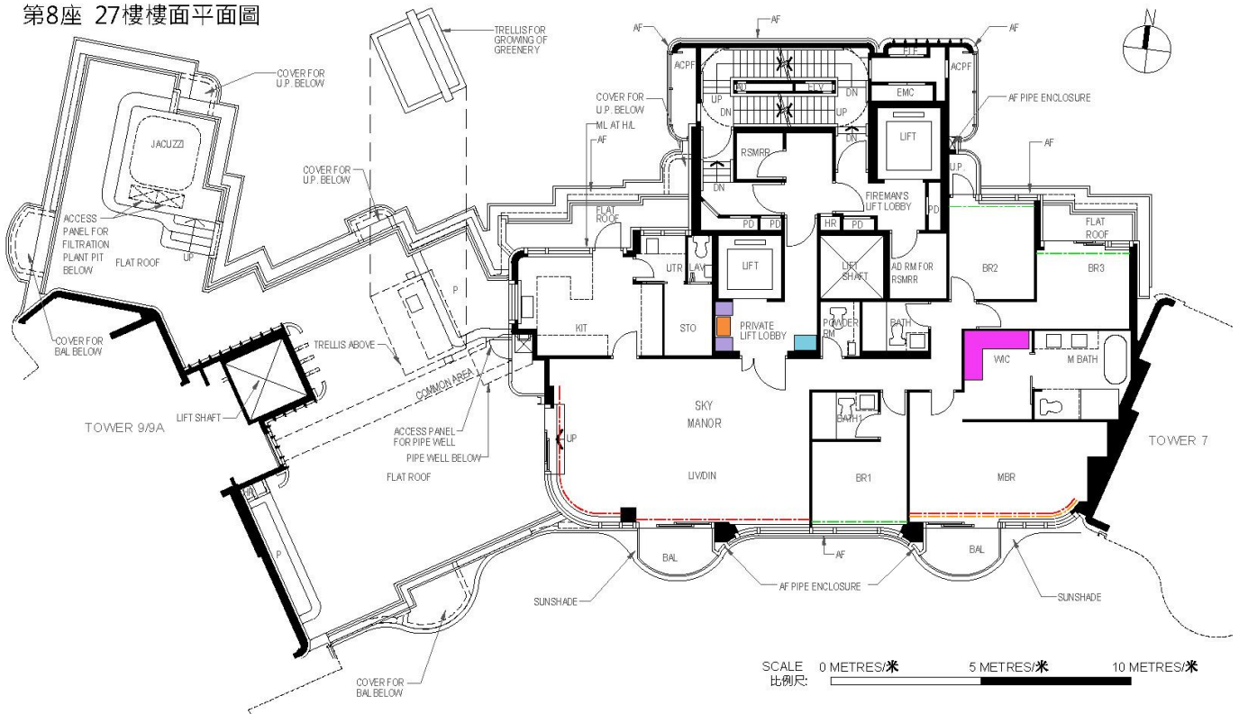
Tower 8 27/F Floor Plan 第8座 27樓樓面平面圖
