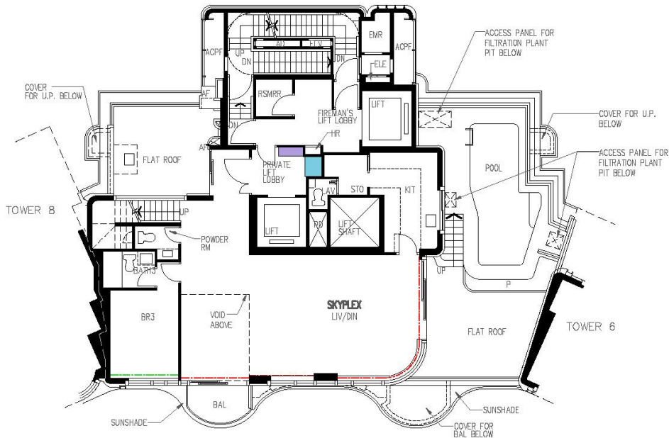
Tower 7 27/F Floor Plan 第7座 27樓樓面平面圖
