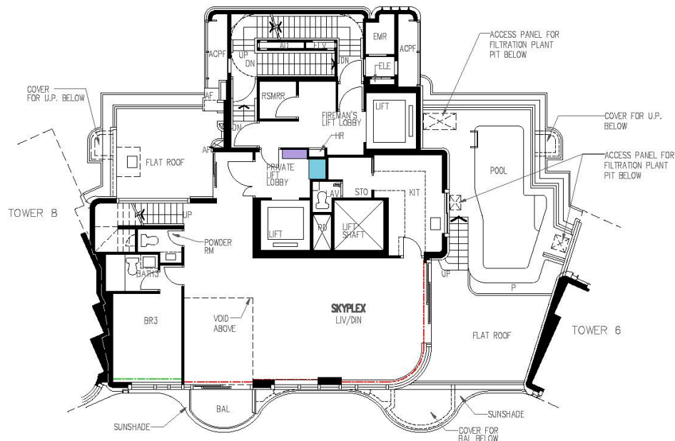
Tower 7 27/F Floor Plan 第7座 27樓樓面平面圖
