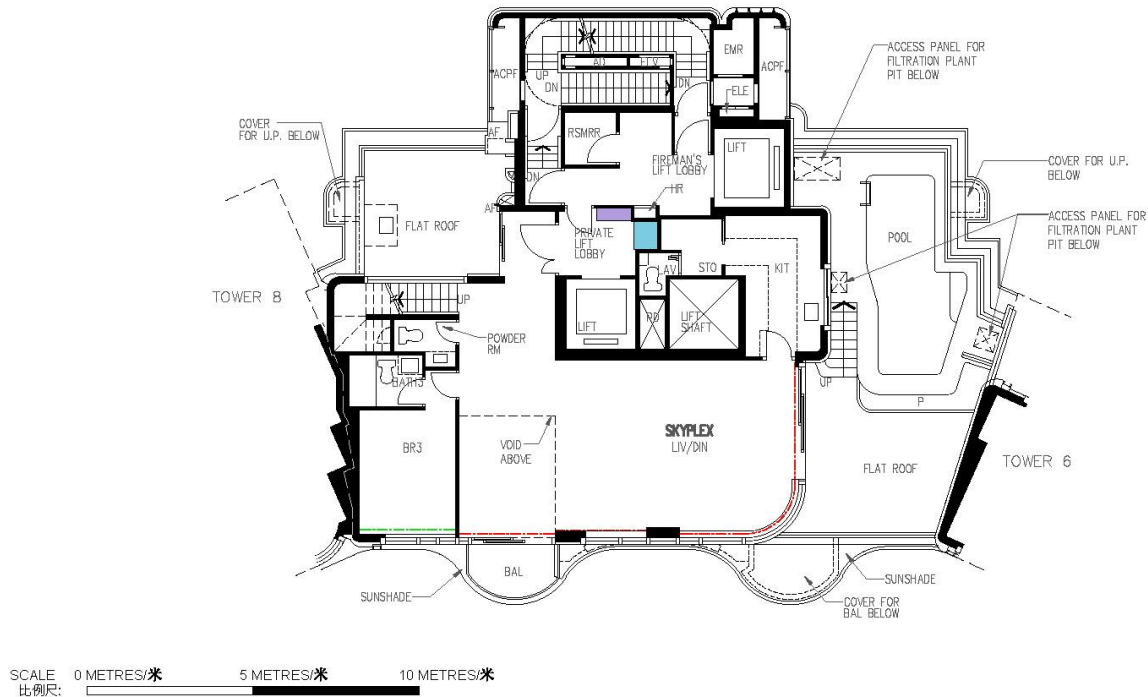
Tower 7 27/F Floor Plan 第7座 27樓樓面平面圖
