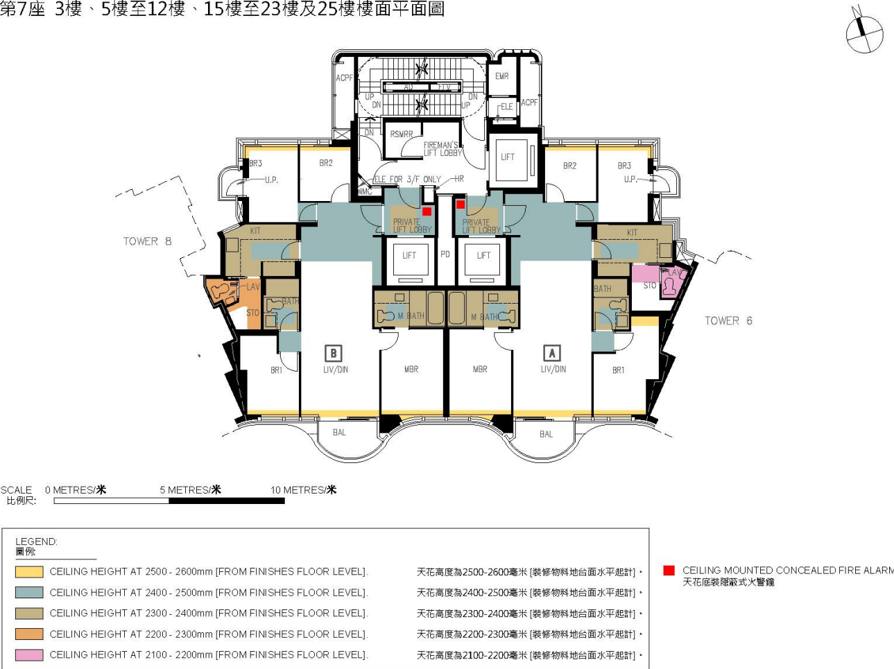
Tower 7 3/F, 5/F-12/F, 15/F-23/F & 25/F Floor Plan 第7座 3樓、5樓至12樓、15樓至23樓及25樓樓面平面圖
