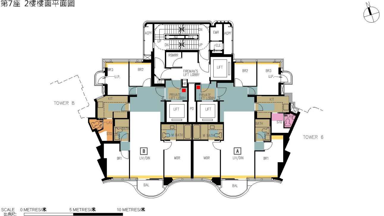
Tower 7 2/F Floor Plan 第7座 2樓樓面平面圖
