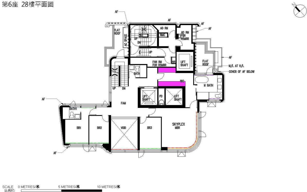
Tower 6 28/F Floor Plan 第6座 28樓平面圖
