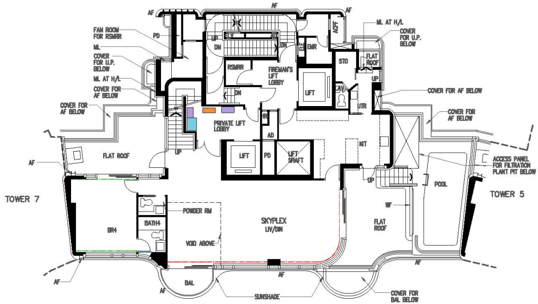
Tower 6 27/F Floor Plan 第6座 27樓平面圖
