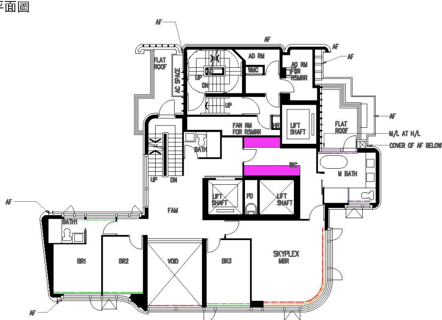
Tower 6 28/F Floor Plan 第6座 28樓平面圖
